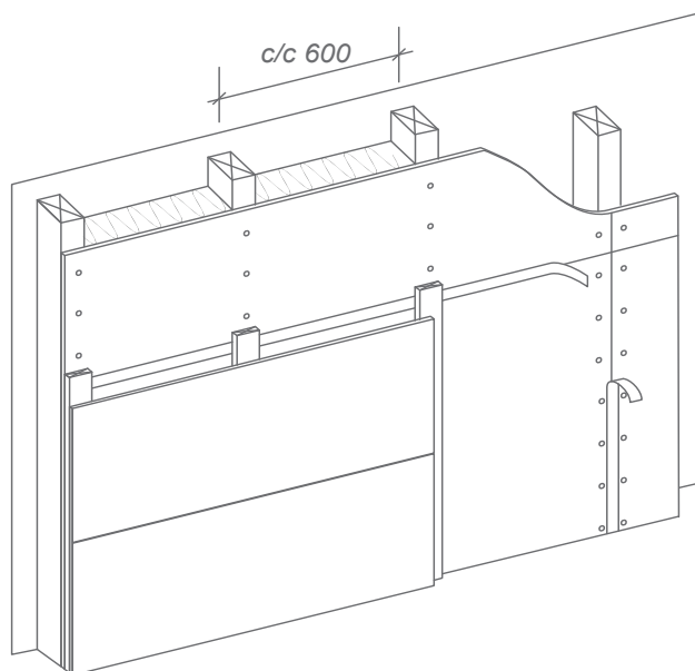
Prinsipp for montering av vindsperreplater for Windpanel Standard og Windpanel Premium.
