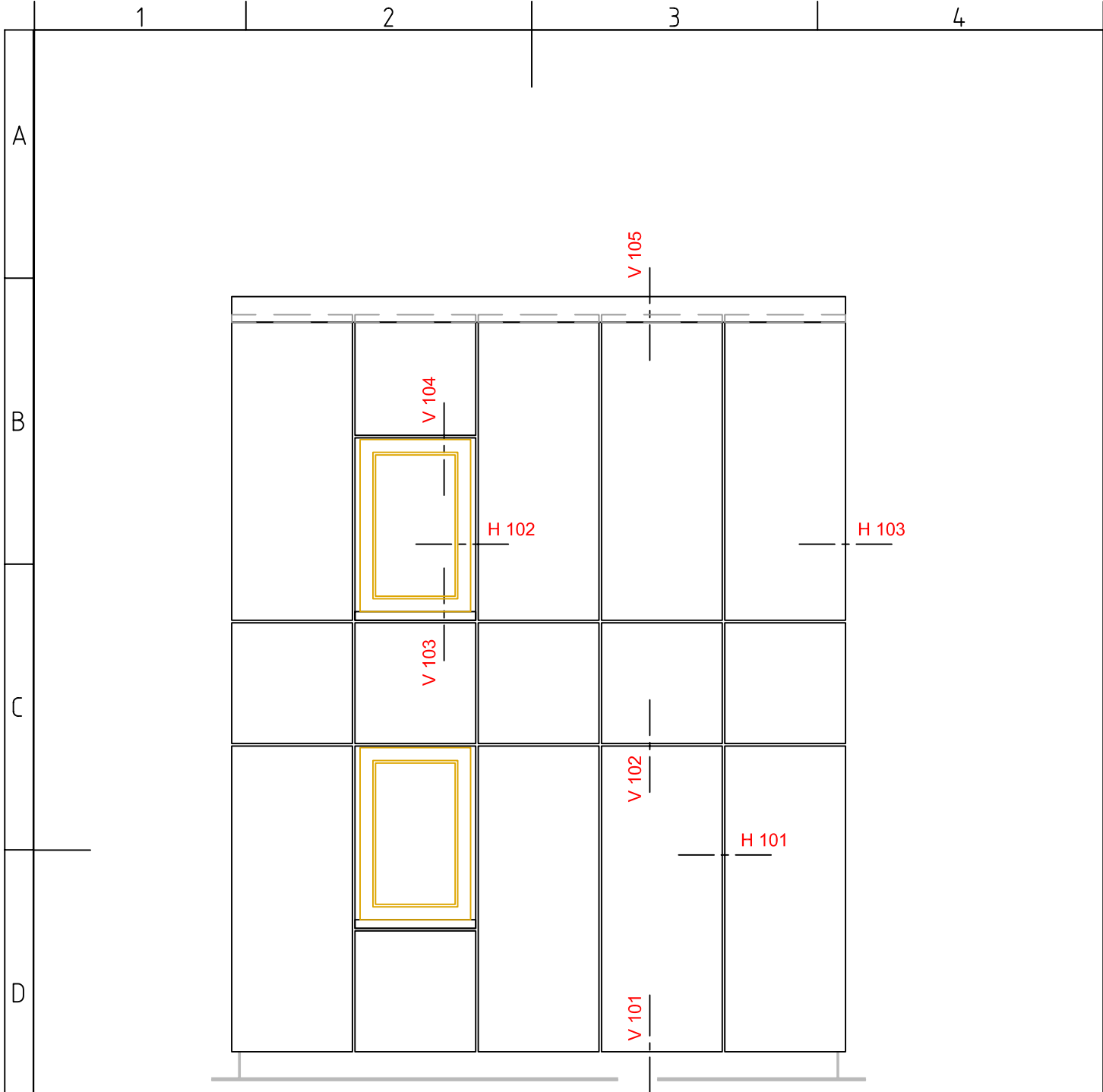
Fassadenansicht / view of cladding
