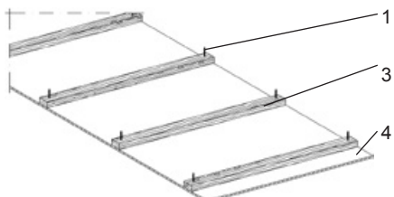
Enkelt trælægtekonstruktion
