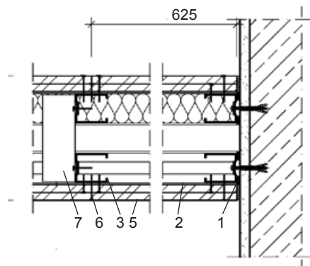
Vandret snit
