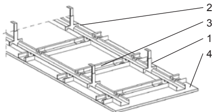
Nedsænket loft med niveauudlignende CD-grund- og bæreprøfil i nonius-nedhængere
