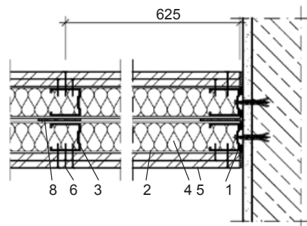
Vandret snit
