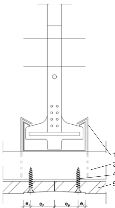
Detalje B Noniusbærer på grundlægger
