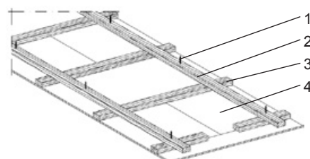
Krydset trælægtekonstruktion
