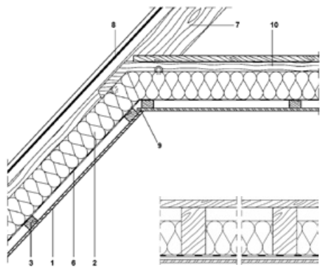
Hydropanel på træ-underkonstruktion Hydropanel på metalunderkonstruktion
