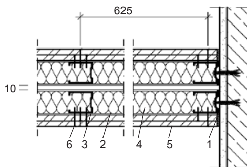
Vandret snit
