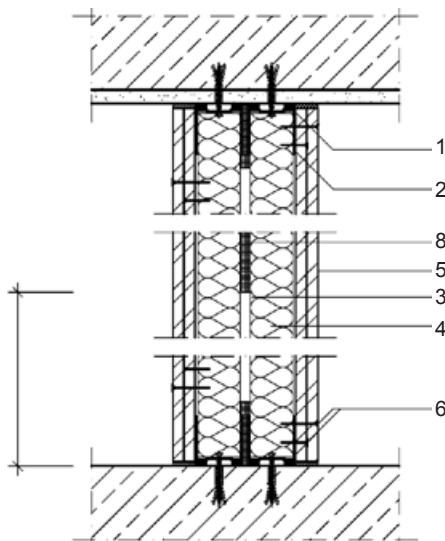
Lodret snit
