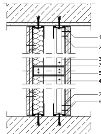
Lodret snit
