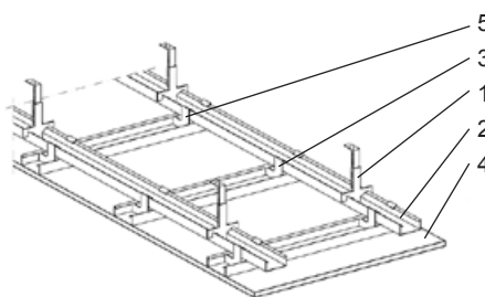
Nedsænket loft med CD-grund- og bæreprøfil i nonius-nedhængere
